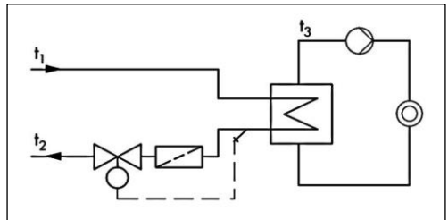
3. Temperature Control of return flow ۳. کنترل دمای جریان برگشتی
