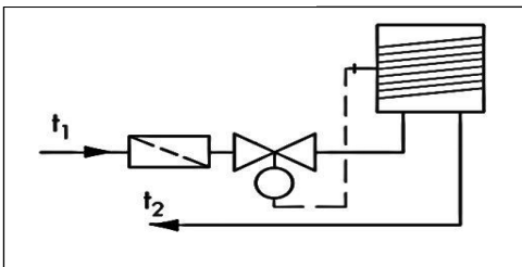
4. Air Temperature Control inside the Air Conditioner ۴. کنترل دمای هوای هواساز
