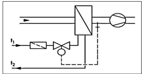
3. Temperature Control of return flow ۳. کنترل دمای جریان برگشتی
