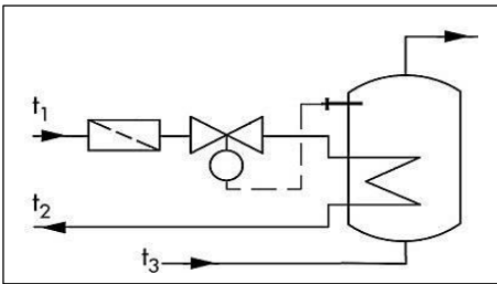
4. Air Temperature Control inside the Air Conditioner ۴. کنترل دمای هوای هواساز
